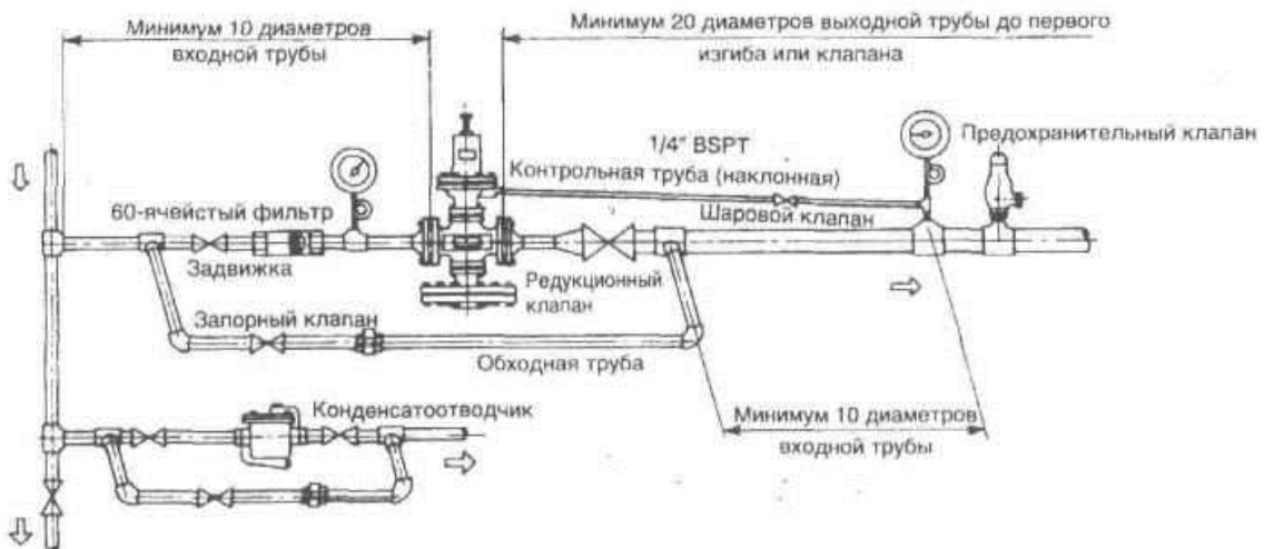
Редуциционная станция – общий вид
